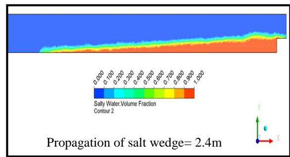
b- Discharge= 55.6 l/min.
