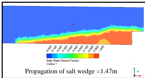
a- Discharge= 45.1 l/min
