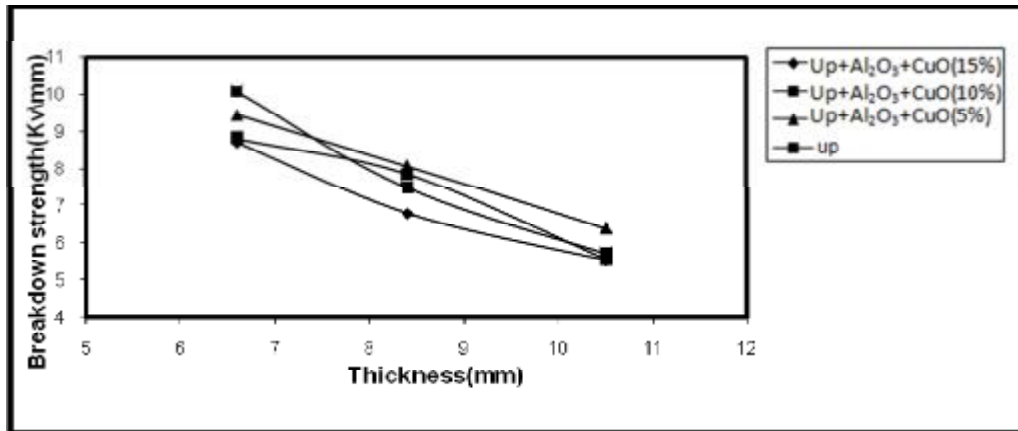
شكل (2) يوضح العلاقة بين متانة العزل والسمك للمترابك الهجين (up+Al 2 O 3 +CuO) وبكسور وزنية مختلفة
