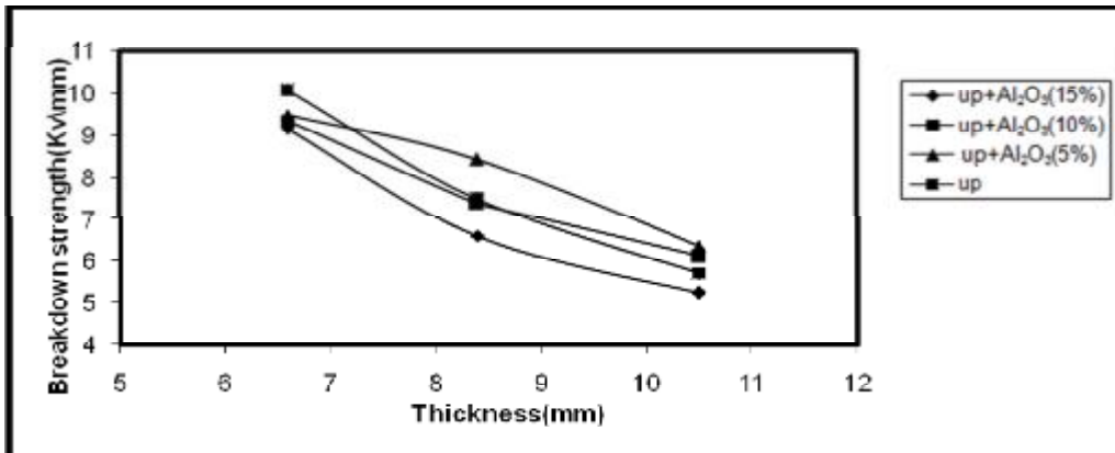
شكل (1) يوضح العلاقة بين متانة العزل والسمك للمتراكبات المنفردة (up+Al 2 O 3 ) وبكسوروزنية مختلفة
