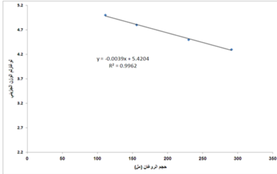
الشكل 3 : المنحني القياسي لتحديد الوزن الجزيئي بتقنية الترشيح الهلامي باستخدام عمود الفصل نوع Sephadex G-50.
