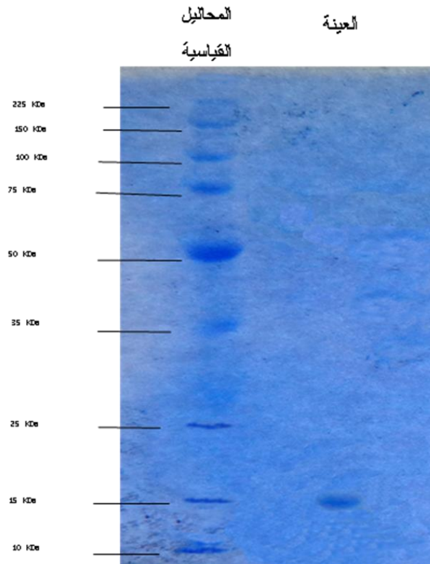
الشكل 4 : يوضح عملية الهجرة الكهربائية لعينة التأثيروروكسين المفصلة من مصل الدم والناتجة من عمود الترشيح الهلامي نوع سيفادكس G-50 مقارنة مع المحاليل القياسية.
