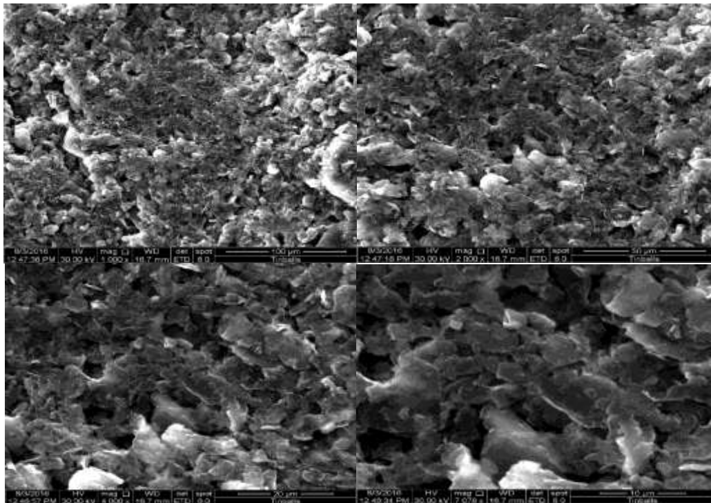
Figure 19- SEM images for (Sol.5).
