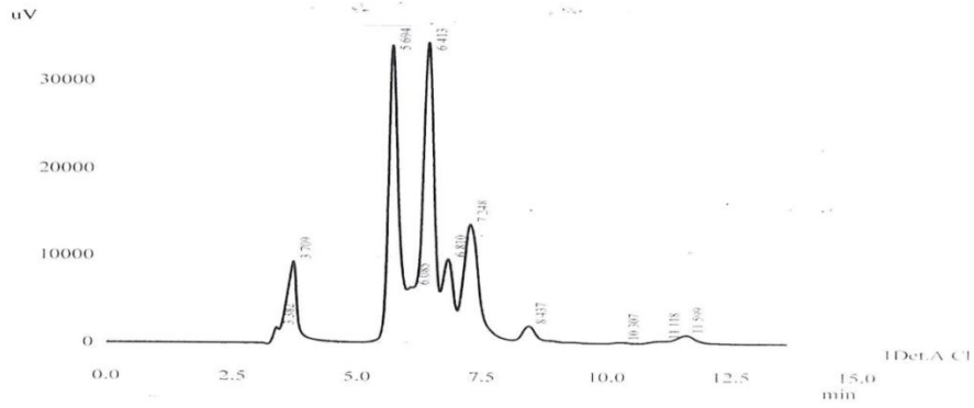
شكل (4) منحنيات مركبي Quercetin و Arctiin في جذور النباتات المزروعة في الموعد الاول والمعاملة بحامض الساليسيليك بتركيز 0 ملغم/لتر -1 (رش ماء فقط)
