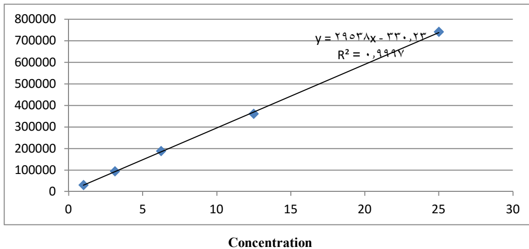
شكل (1) المخطط القياسي لمركب Quercetin
