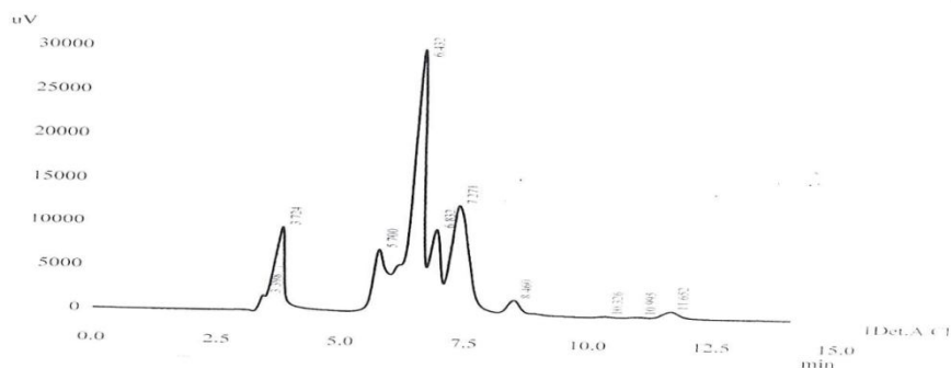
شكل (5) منحنيات مركبي Quercetin و Arctiin في جذور النباتات المزروعة في الموعد الثالث والمعاملة بحامض الساليسيليك بتركيز 200 ملغم.لتر -1
