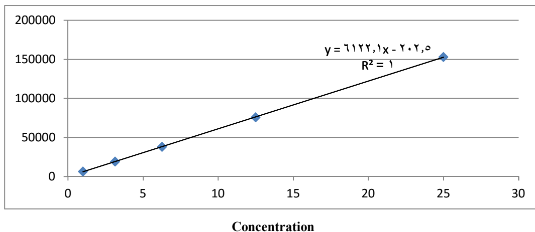
شكل (2) المخطط القياسي لمركب Arctiin
