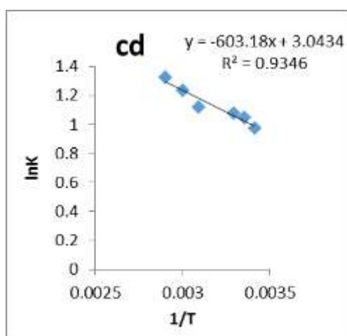
Figure(8)Vant Huff curve (Cd)
