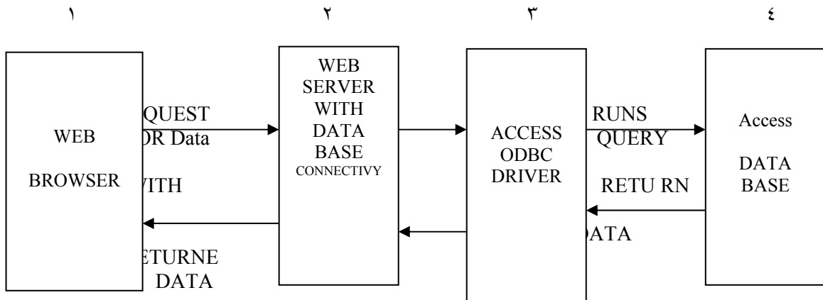
الشكل (٢-٢) يوضح ترابط قواعد بيانات نظام الموقع المصدر : ( Ian Somerville software Engineering : ١٩٩٥ )
