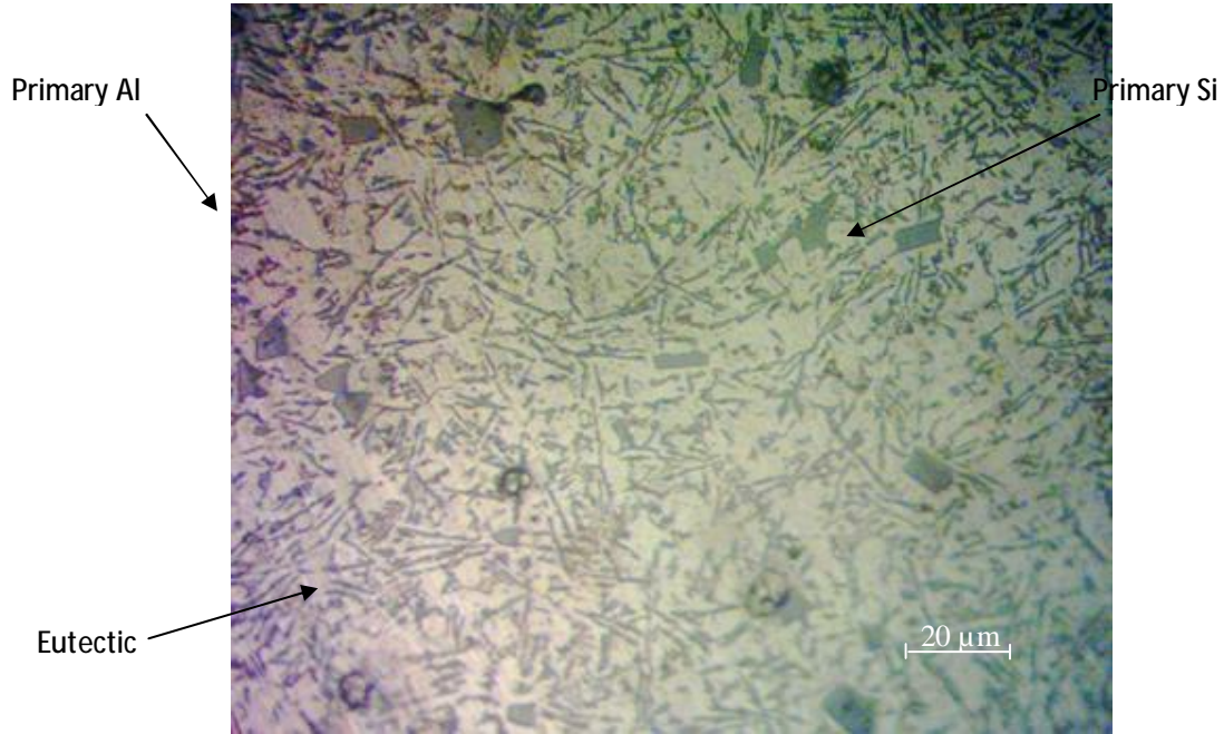
الشكل رقم (1): البنية المجهرية لسبيكة (Al-14%Si) المصبوبة
