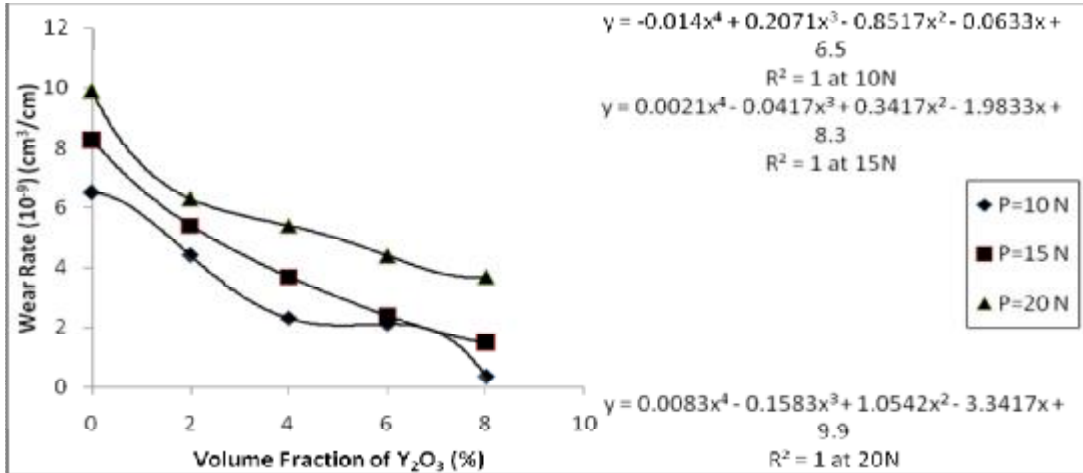
الشكل رقم (7) علاقة معدل البلى مع الكسر الحجمي للمواد المترابطة عند زمن (5) دقائق
