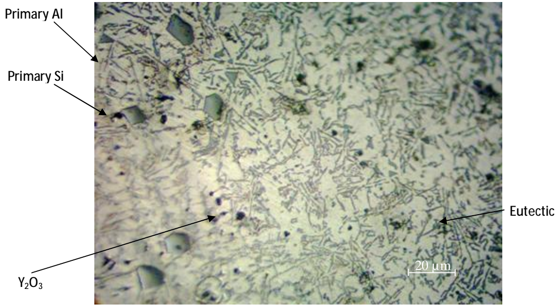
الشكل رقم (4): البنية المجهرية للمادة المترابطة (6% Y_2O_3 /Al-14%Si)
