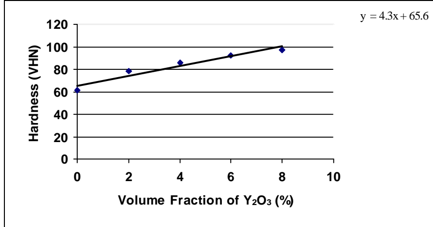
الشكل رقم (6) علاقة الصلادة مع الكسر الحجمي لدقائق الايتريا في المواد المترابطة
