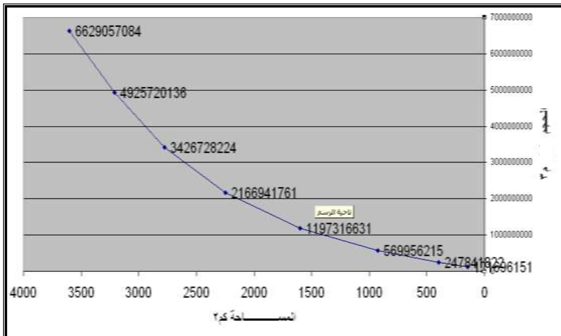
الشكل (6) العلاقة بين المساحة السطحية للمياه (كم 2 ) وحجم المياه الممكن خزنها في الهور (م 3 )
