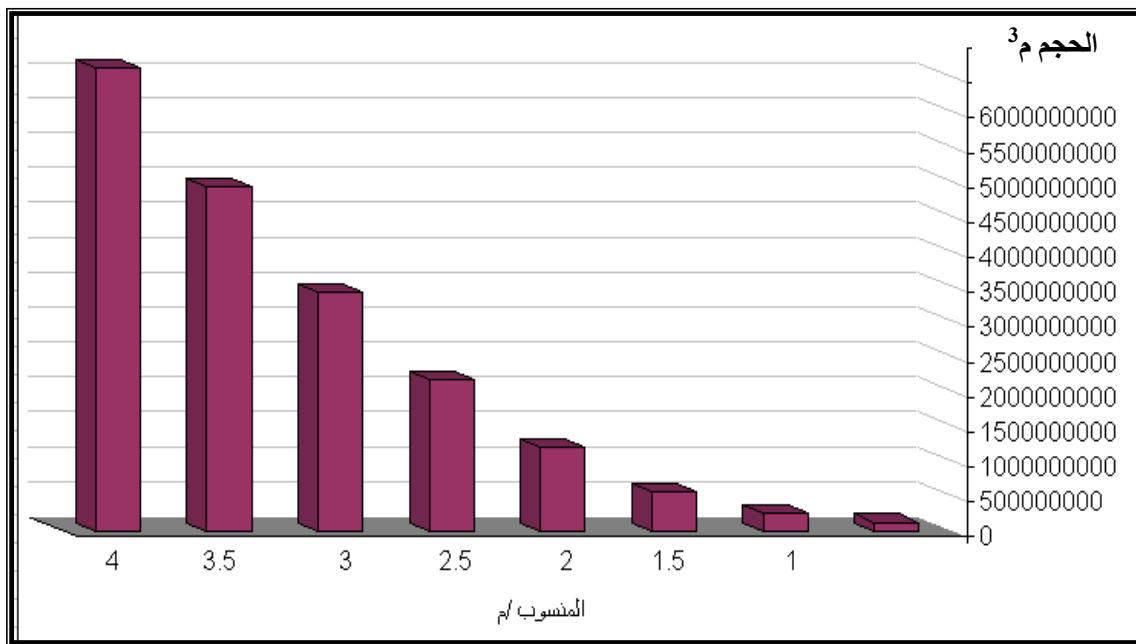
شكل (5) العلاقة بين منسوب الماء (م) في الهور وحجم المياه الممكن خزنها فيه (م 3 )
