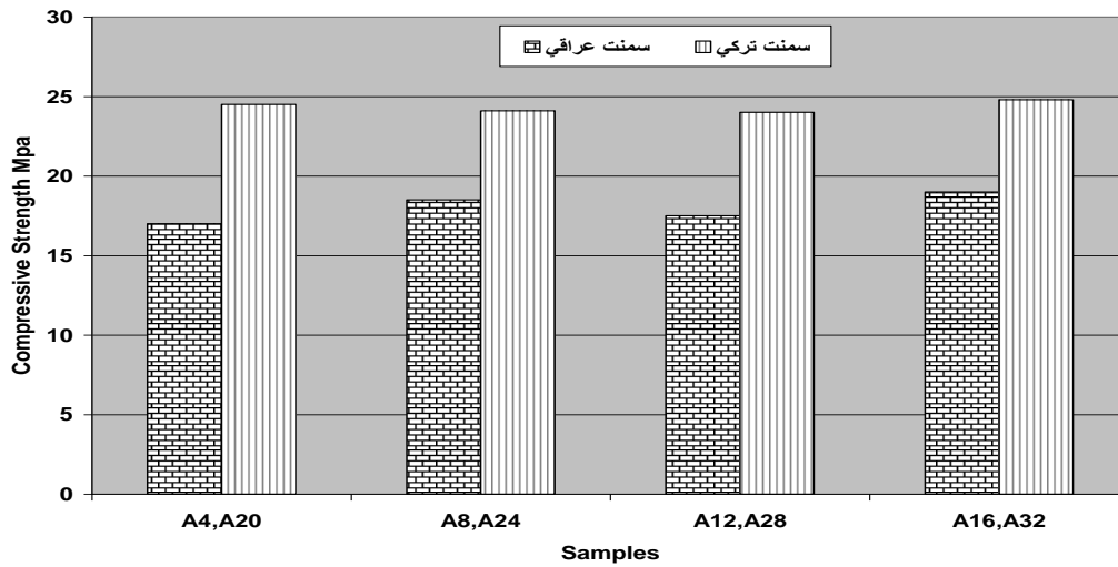
شكل (11) يوضح تأثير نوع السمنت على قابلية التحمل للمكعبات الخرسانية بعمر 28 يوم
