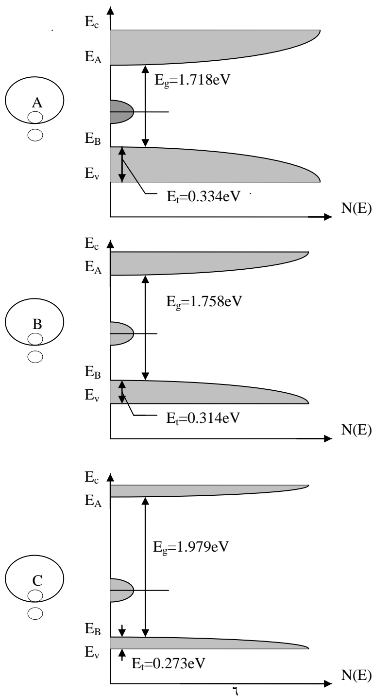
الشكل (9): مخطط كثافة الحالات لغشاء \text{CuIn}(\text{Se}_{0.4}\text{Te}_{0.6})_2 الرقيق قبل التلدين.
