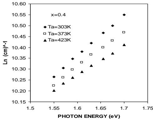
الشكل (8): تغيير عرض الذبول مع طاقة الفوتون لغشاء CuIn(Se_{0.4}Te_{0.6})_2 الرقيق قبل التلدين وبعده.
