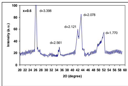
الشكل(2): طيف حيود الاشعة السينية للمركب \text{CuIn}(\text{Se}_{0.6}\text{Te}_{0.4})_2
