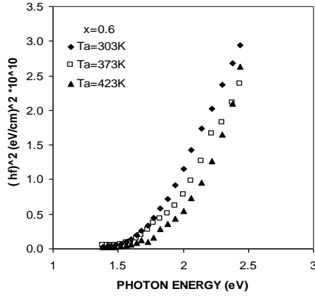
الشكل (5): تغير فجوة الطاقة مع طاقة الفوتون لعشاء \text{CuIn}(\text{Se}_{0.6}\text{Te}_{0.4})_2 الرقيق قبل التلدين وبعده.
