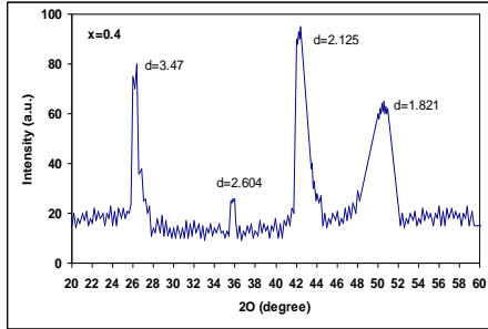
الشكل(1): طيف حيود الاشعة السينية للمركب \text{CuIn}(\text{Se}_{0.4}\text{Te}_{0.6})_2
