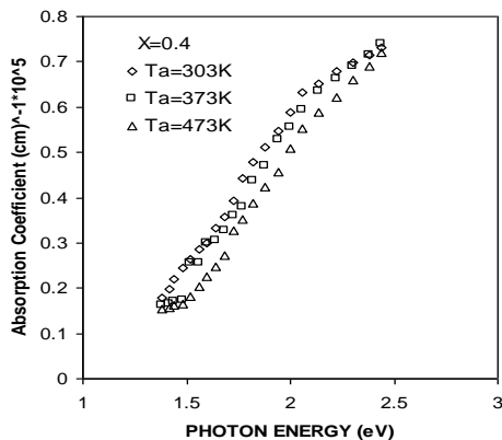
الشكل (4): تغير معامل الامتصاص مع طاقة الفوتون لغشاء CuIn(Se_{0.4}Te_{0.6})_2 الرقيق عند درجات تليدين مختلفة.
