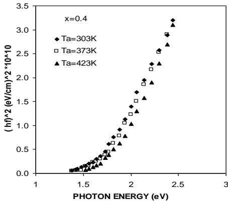
الشكل (5): تغير فجوة الطاقة مع طاقة الفوتون لعشاء \text{CuIn}(\text{Se}_{0.6}\text{Te}_{0.4})_2 الرقيق قبل التلدين وبعده.
