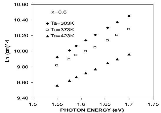
الشكل (7): تغيير عرض الذبول مع طاقة الفوتون لغشاء CuIn(Se_{0.6}Te_{0.4})_2 الرقيق قبل التلدين وبعده.
