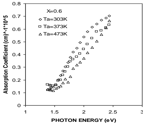
الشكل (3): تغير معامل الامتصاص مع طاقة الفوتون لغشاء CuIn(Se_{0.6}Te_{0.4})_2 الرقيق عند درجات تليدين مختلفة.
