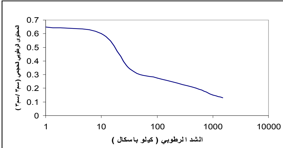
شكل-1: منحنى الوصف الرطوبي لتربة الحقل
