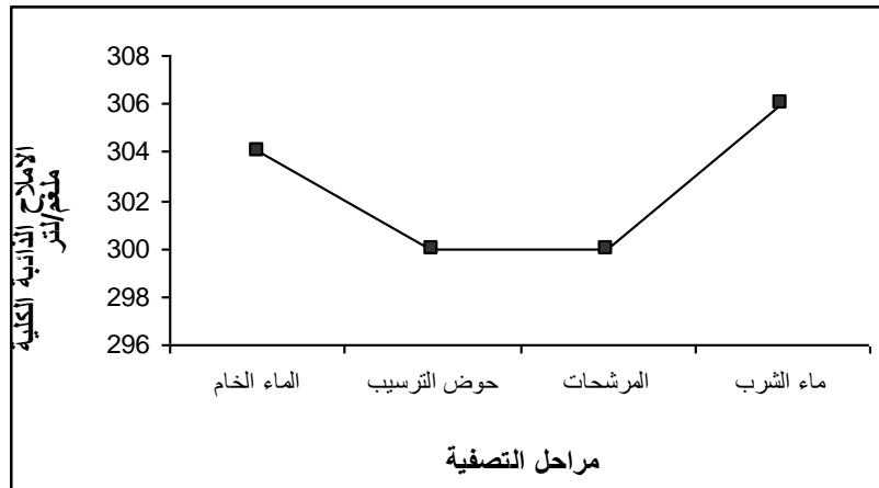
شكل رقم (6) معدل قياس الـ TDS في مراحل الصفية
