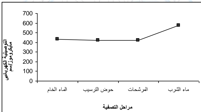
شكل رقم (7) معدل قياس التوصيلية الكهربائية في مراحل الصفية
