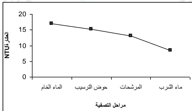
شكل رقم (5) معدل قياس العكارة في مراحل التصفية
