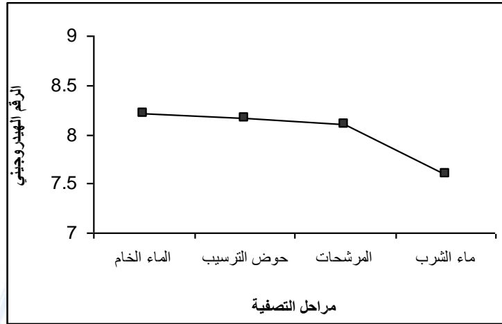
شكل رقم (4) معدل قياس الرقم الهيدروجيني في مراحل التصفية
