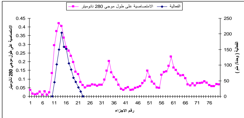
شكل (1) كروماتوغرافيا التبادل الايوني باستخدام عمود المبادل الهيمولايسين ، بسرعة جريان 20 مل /ساعة وبواقع 5 مل / جزء. 12x3 سم لتنقية انزيم DEAE-cellulose بابعاد سم لتنقية انزيم
