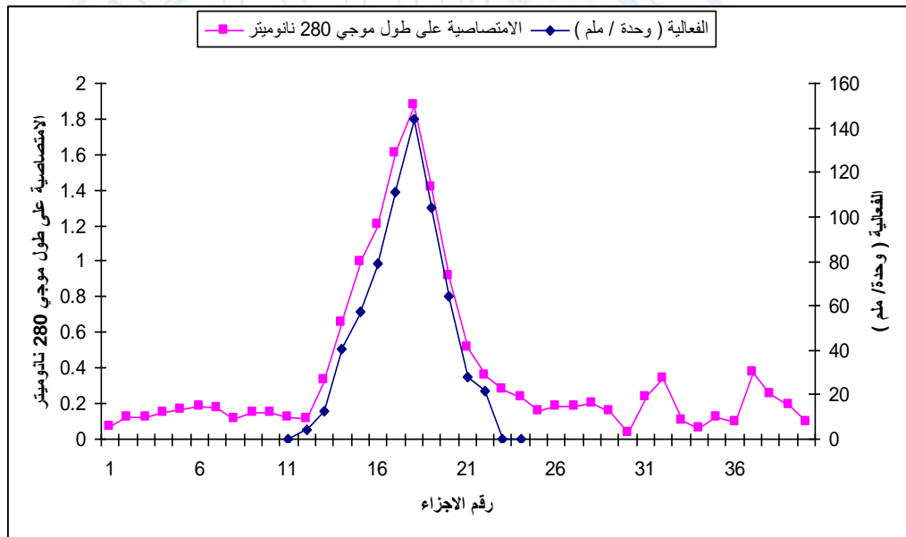
الشكل(2) كروماتوغرافيا الترشيح الهلامي للهيمولايسين باستخدام عمود الترشيح الهلامي Sephadex-G100 بابعاد 35X1.5 سم . تم الغسل بمحلول 0.2 مولار من دارى الفوسفات ذي رقم هيدروجيني 7.5 وبسرعة جريان 12 مل/ساعة وبواقع 4 مل / ساعة.
