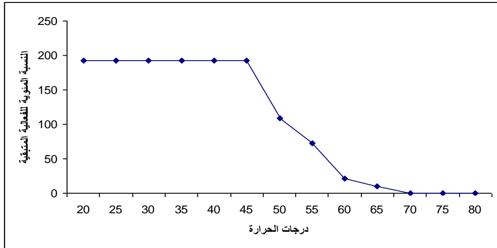
الشكل (7) الثبات الحراري للهيمولايسين المنقى من العزلة المحلية لبكتريا الهيضة بتعرضها لدرجات حرارة مختلفة ( 80 - 20 ) م
