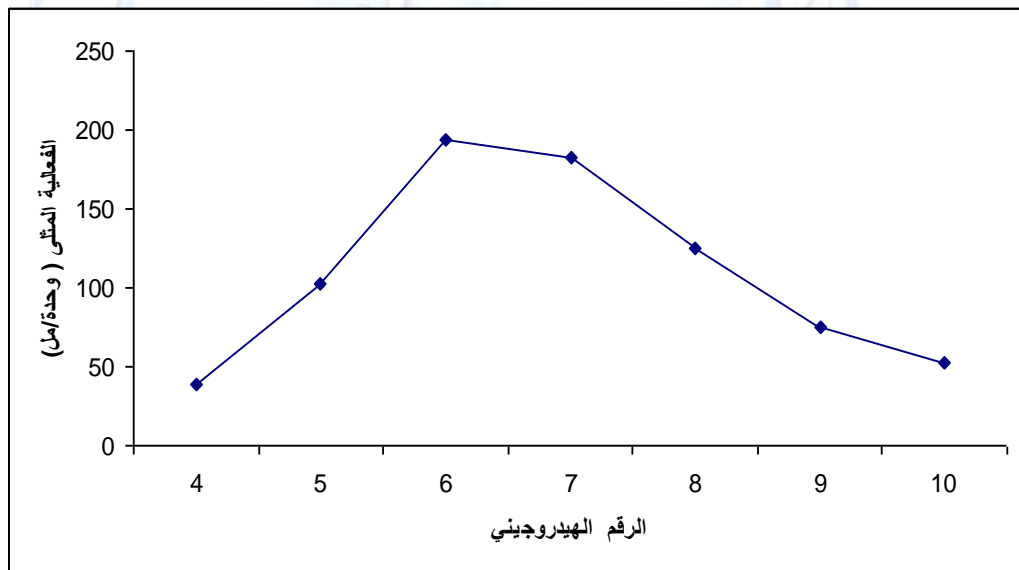
الشكل (4) تأثير قيم مختلفة من الرقم الهيدروجيني (4-10) في فعالية الهيمولايسين المنقى من العزلة المحلية لبكتريا الهيضة
