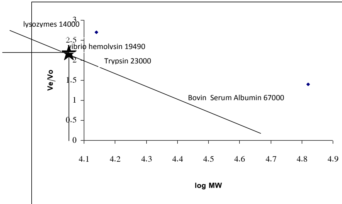
الشكل (3) تحديد الوزن الجزيئي للهيمولايسين المنتج من العزلة المحلية لبكتريا الهيضة باستخدام الترشيح الهلامي
