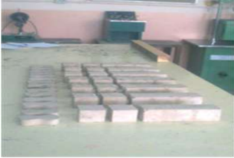
صوره رقم(5): بعض نماذج مونة الجص للضغط والشد ومعايير الكسر
